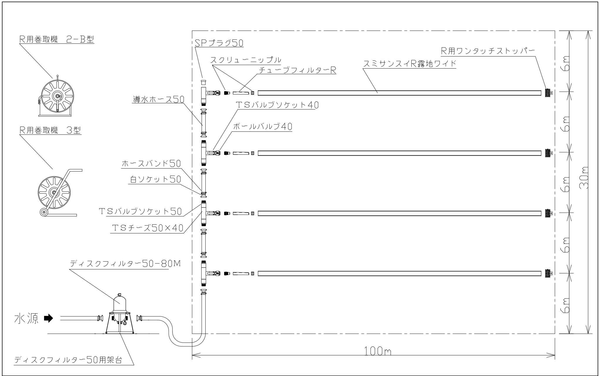
スミサンスイR露地ワイド 配管例 (30a)
