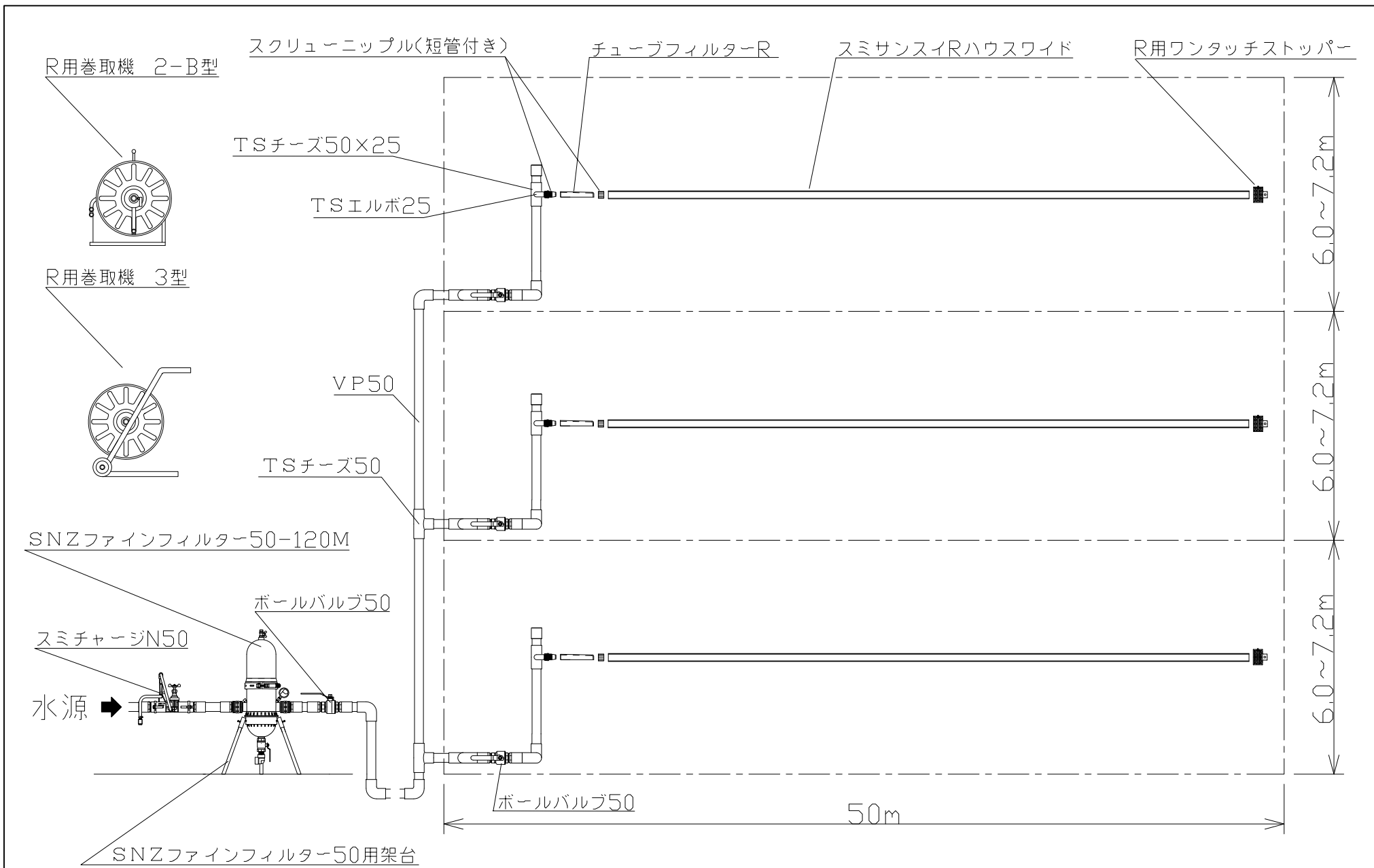
スミスンスイRハウスイド 配管例(10a)
