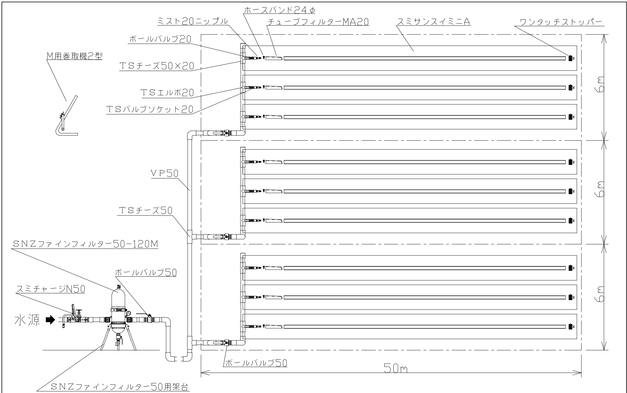
スミサンスイミニA 配管例 (10a)
