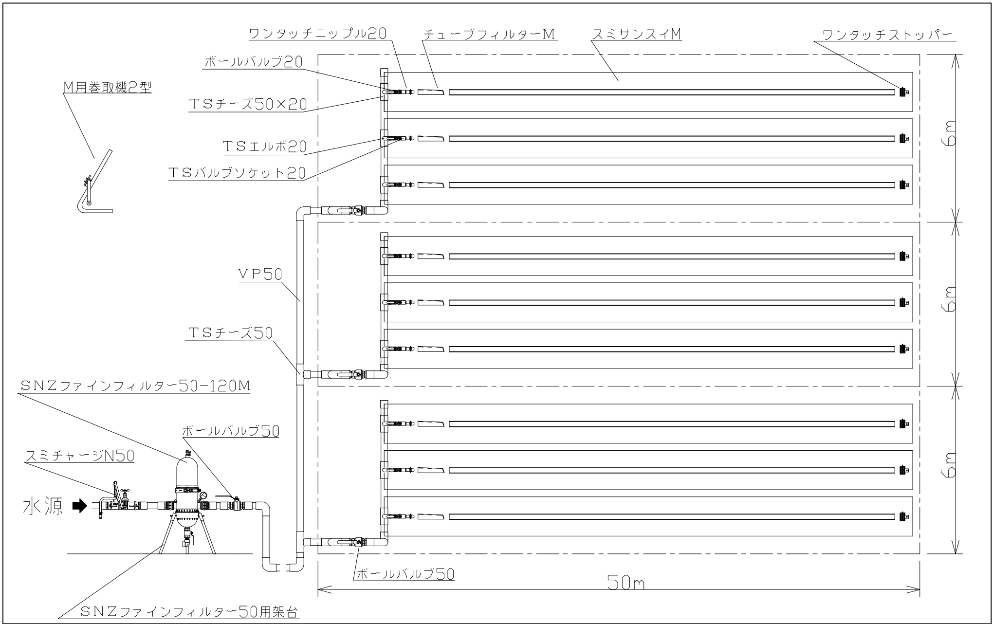
スミサンスイM 配管例(10a)
