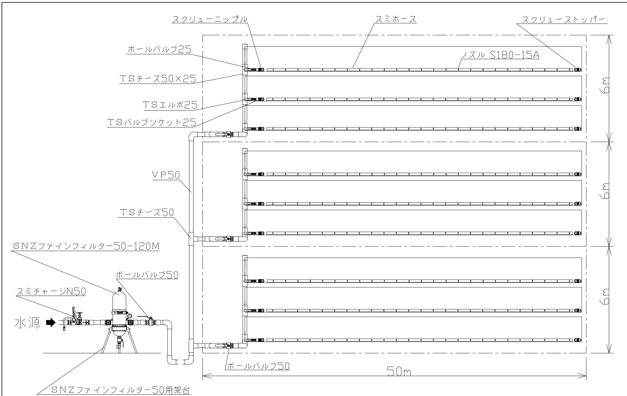
スミホース ノズル：S180-15A 配管例（10a）
